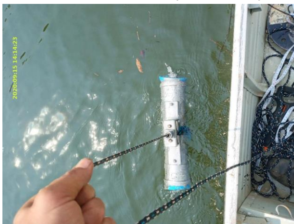
Garrafa de Van Dorn (Coleta MQA)
