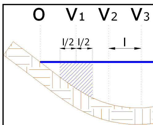
Figura 2 – Delimitação da sub-seção da vertical 1
