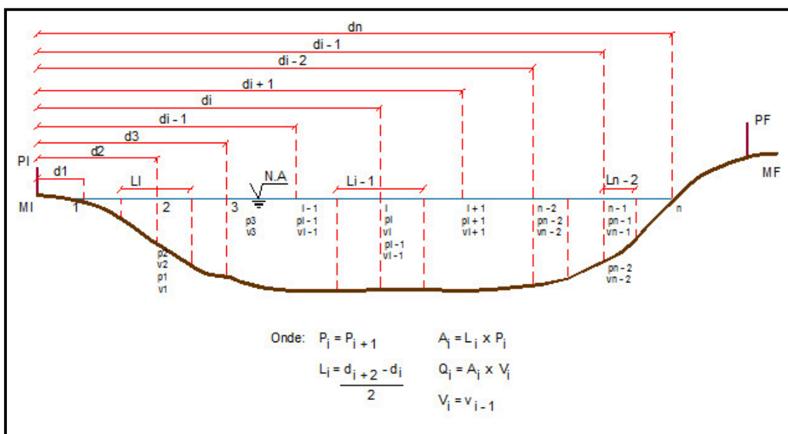
Figura 4 – Croqui do método da meia seção considerando fórmula da área de um trapézio
