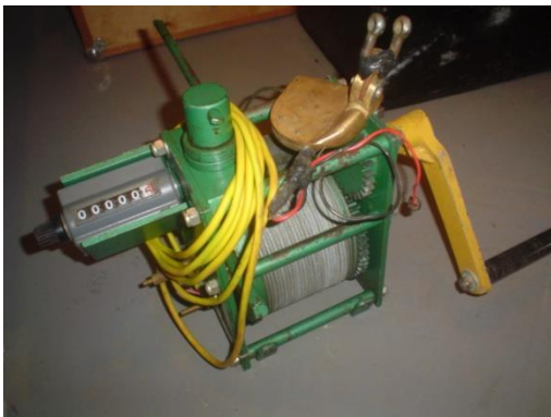
Guincho Hidrométrico
